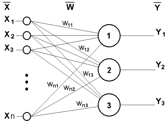
Рис.3. Однослойный перцептрон
