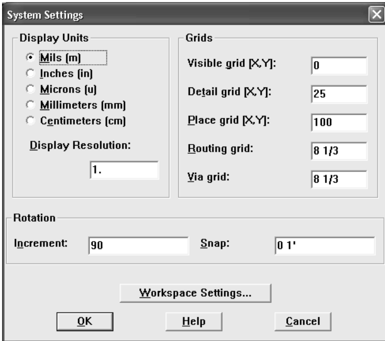
Рис. 8. Редактирование параметров проекта
