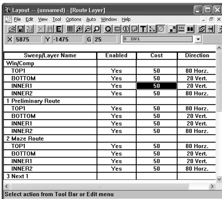
Рис. 9. Конфигурирование слоев ПП
