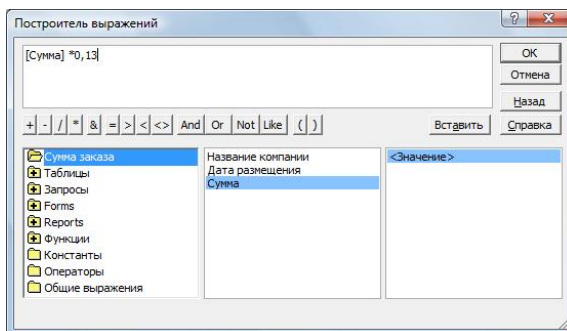
Рис. 8. Построитель выражений
