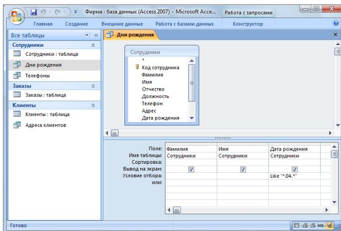
Рис. 5. Создание запроса
