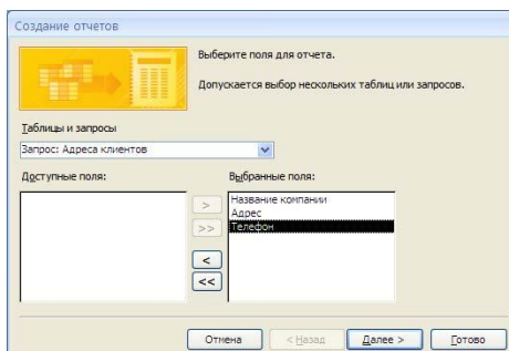
Рис. 15. Мастер отчетов
