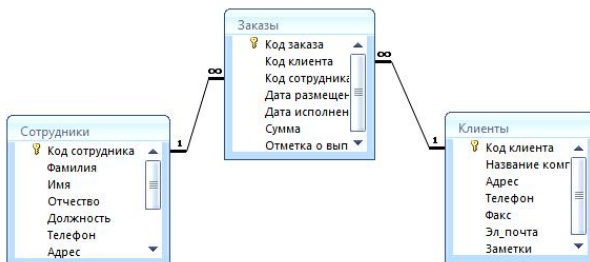
Рис. 2. Схема данных
