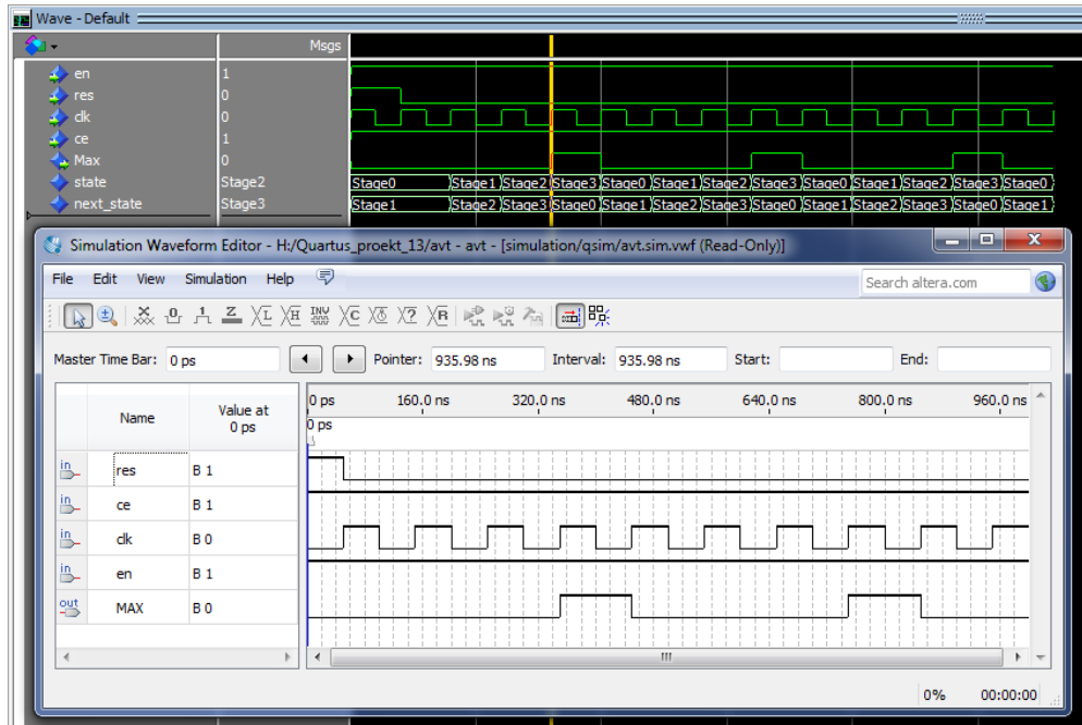
Рис. 9. Функциональное моделирование конечного автомата в ModelSim Altera Started Edition и в векторном редакторе САПР Altera Quartus II
