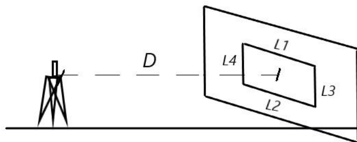
Рис. 6.1. Схема калибровки съёмочной камеры
