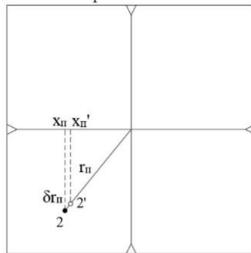
Рис. 1.3. Схема определения плановых смещений на снимках
