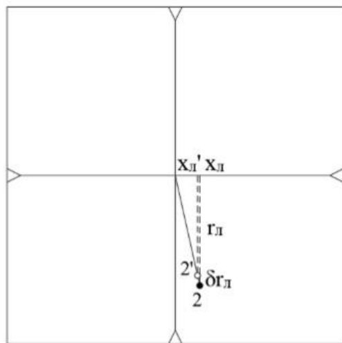
Рис. 1.3. Схема определения плановых смещений на снимках
