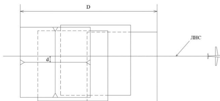
Рис. 3.3. Определение не прямолинейности маршрута
