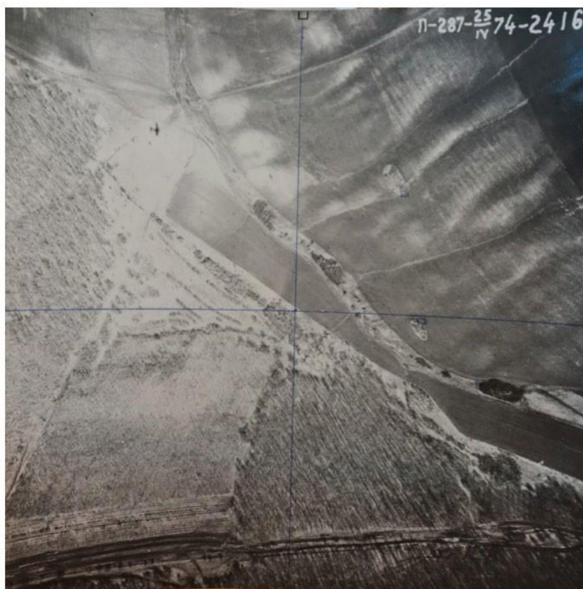
Рис. 4.1. Снимок местности.
