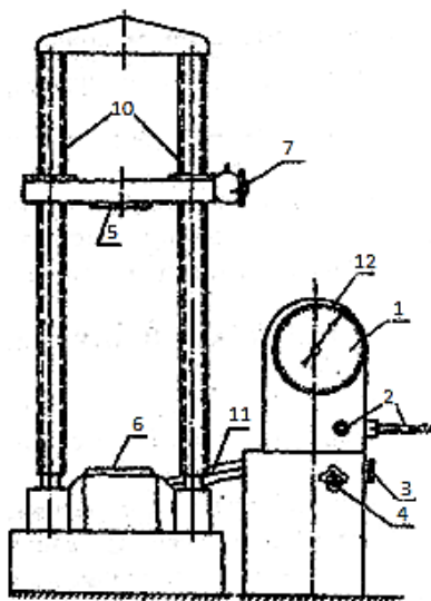
Рис. 2.3. Эскиз пресса гидравлического 2ПГ-250
