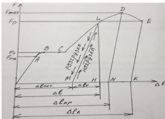
Рис. 1.5. Диаграмма растяжения малоуглеродистой стали
