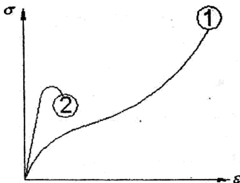
Рис. 2.2. Диаграммы сжатия: 1-пластичного материала, 2-хрупкого материала
