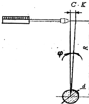
Рис. 3.3. Схема для определения абсолютного угла закручивания
