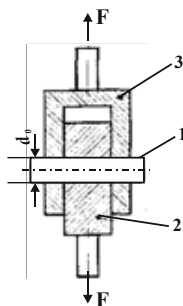
Рис.5.1 Эскиз приспособления на срез
