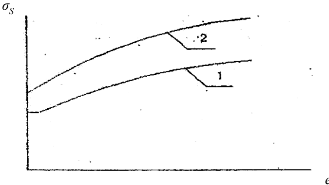
Рис. 2.1. Кривые упрочнения малоуглеродистой и легированной сталей
