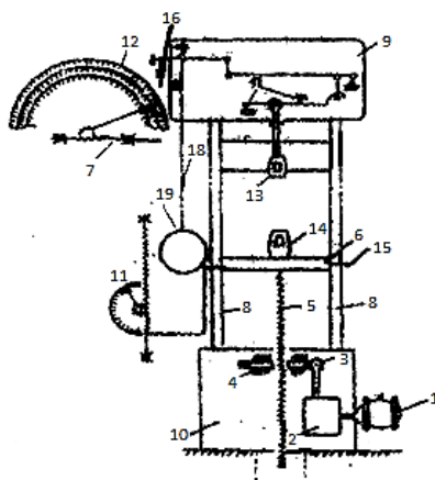
Рис. 1.6. Эскиз испытательной машины УМ - 5
