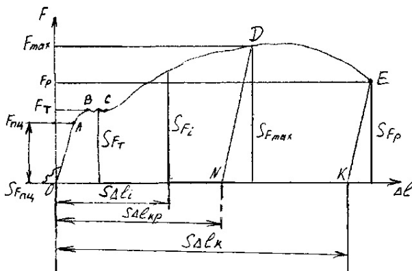
Рис. 1.7. Характерные точки диаграммы растяжения
