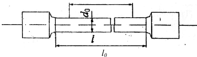
Рис. 1.1. Образец для испытания на растяжение
