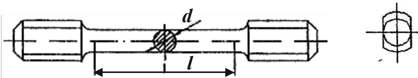
Рис. 3.1. Образец для испытания на кручение
