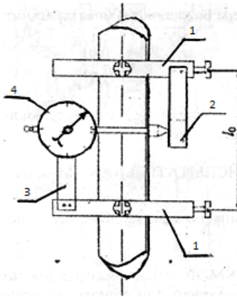
Рис. 3.2. Эскиз приспособления для испытания на кручение
