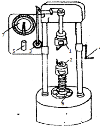
Рис. 3.4. Эскиз испытательной машины на кручение КМ - 50
