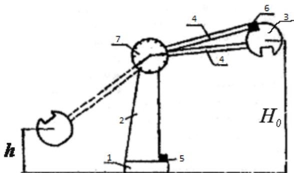
Рис. 4.3. Эскиз маятникового копра МК - 30
