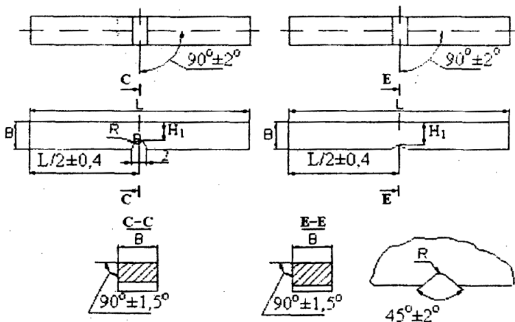
Рис. 4.1. Образец с U надрезом
