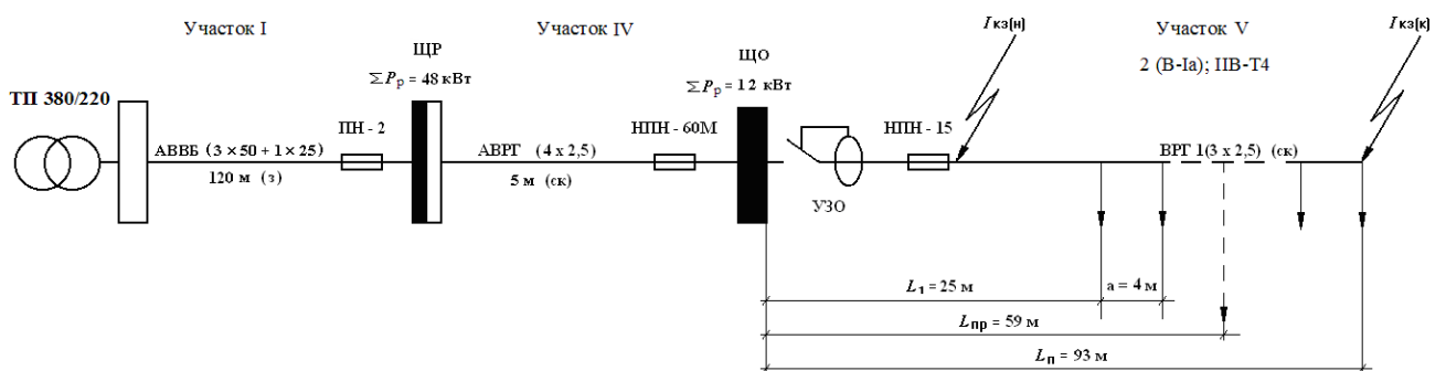
Рис. 3. Расчетная схема силовой сети (защита автоматическими выключателями на участках I, II и III)
