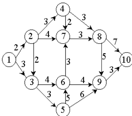
Рис. 1. Сетевой график
