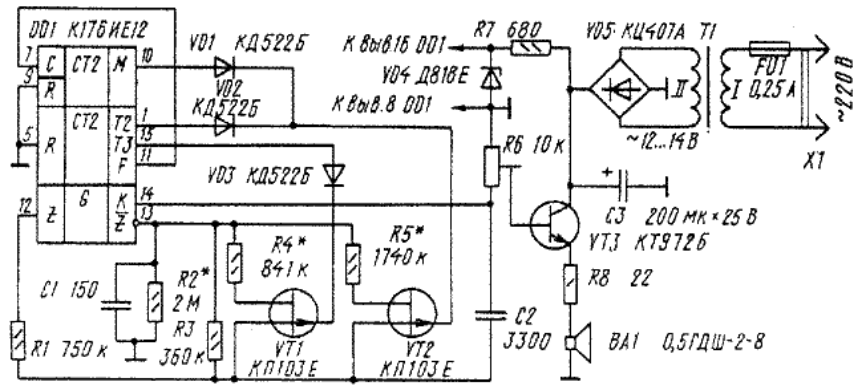
Рисунок 3 – Звонок электронный на микросхеме K176IE12 Вариант №4. Переключатель светодиодных гирлянд
