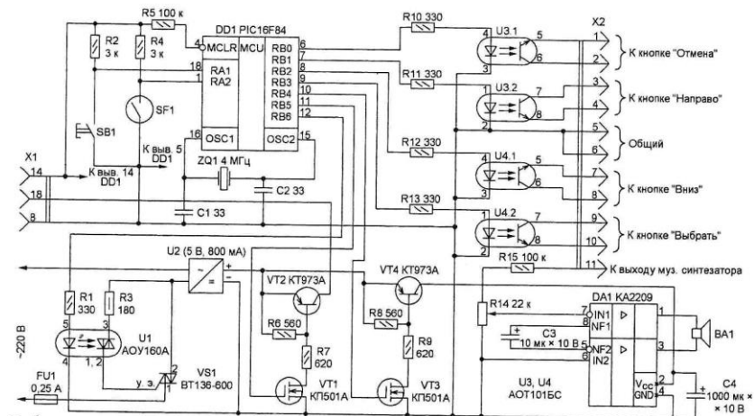
Рисунок 5 – Полифонический квартирный звонок
