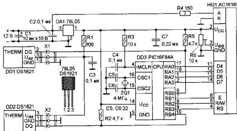
Рисунок 11 – Термометр на DS1821 и PIC-контроллере
