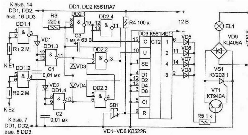
Рисунок 7 – Сенсорный выключатель
