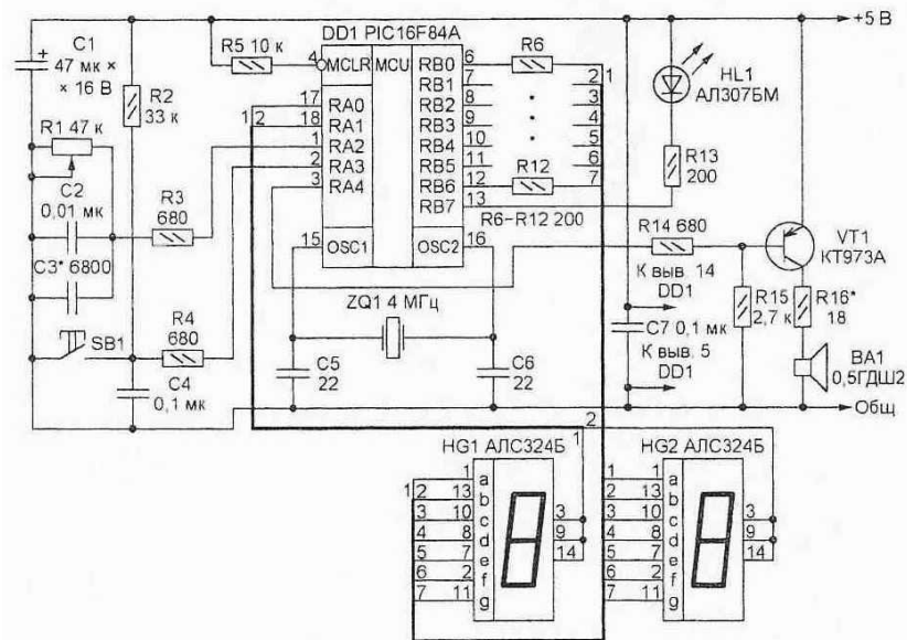
Рисунок 10 – Таймер PIC16F84
