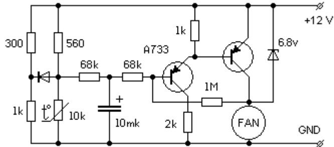
Рисунок 6 - Принципиальная схема регулятора
