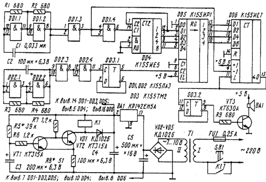
Рисунок 2 - Звонок электронный мелодичный Вариант №3. Звонок электронный на микросхеме K176IE12
