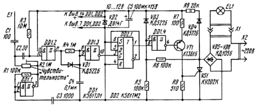
Рисунок 8 - Сенсорный выключатель светильника
