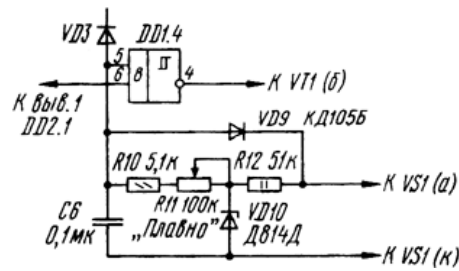
Рисунок 8.1 – Часть узла управления транзистором
