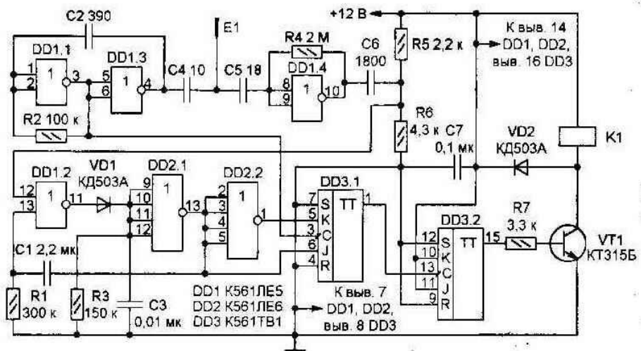
Рисунок 9 – Сенсорный выключатель электронной лампы
