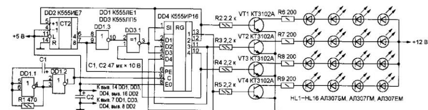
Рисунок 4. – Переключатель светодиодных гирлянд
