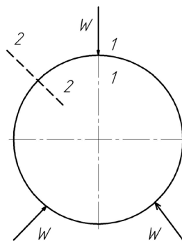
Рис. 1.2. Схема закрепления кольца в трехкулачковом патроне
