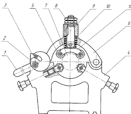
Рис. 2.16. Неподвижный универсальный люнет
