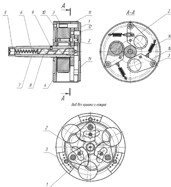
Рис. 2.11. Трехкулачковый поводковый самозажимной патрон
