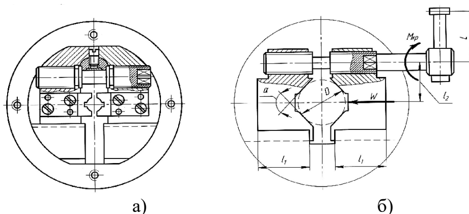
Рис. 2.1. Универсальный двухкулачковый самоцентрирующий патрон с ручным винтовым зажимом: а) конструктивная схема; б) расчетная схема
