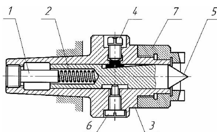
Рис. 2.9. Поводковая оправка: 1–упорный винт; 2–пружина; 3– корпус; 4– стопорный винт; 5–подпружиненный (плавающий) центр; 6– винт; 7– зубья/штырьки
