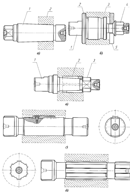
Рис. 2.17. Типы жестких центровых оправок
