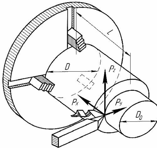
Рис. 2.2. Расчетная схема токарного патрона
