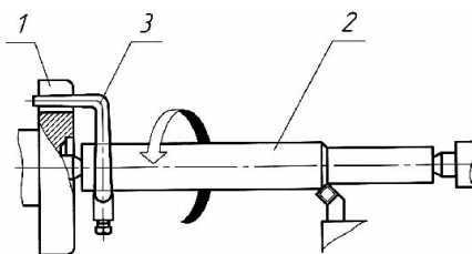
Рис. 2.7. Заготовка инструмента, установленная в центрах: 1– планшайба; 2– заготовка инструмента; 3– хомутик
