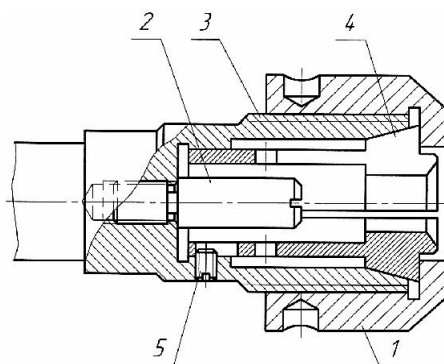
Рис. 2.4. Универсальный цанговый патрон: 1– нажимная гайка; 2– регулируемый упор; 3– корпус; 4– цанга; 5– винт. 4.3
