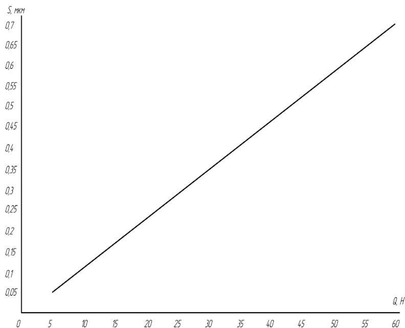
Рис. 1.4. Тарировочный график динамометрического ключа
