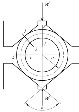
Рис. 1.3. Схема закрепления кольца в призму
