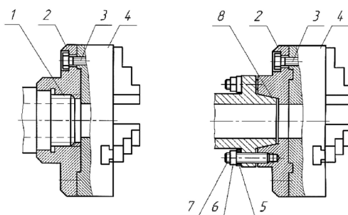
Рис. 2.3. Закрепление токарного патрона на шпинделе станка: 1– резьбовой конец шпинделя; 2– планшайба; 3– винт; 4– корпус; 5– шайба; 6– гайка; 7– шпилька; 8– посадочный конус шпинделя
