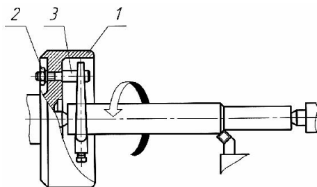
Рис. 2.8. Безопасная планшайба: 1– планшайба; 2– гайка; 3– палец
