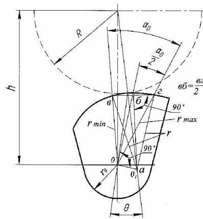
Рис. 2.12. Расчетная схема для определения размеров и профиля кулачков поводковых самозажимных патронов
