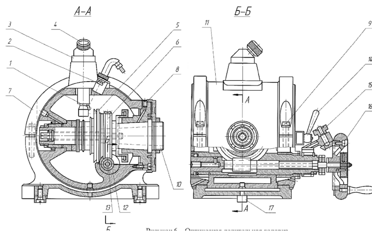
Рис. 3.3. Оптическая делительная головка
