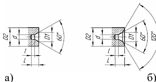
Рис. 2.5. Размеры центровых отверстий: а) тип А без предохранительного конуса; б) тип Б с предохранительным конусом
