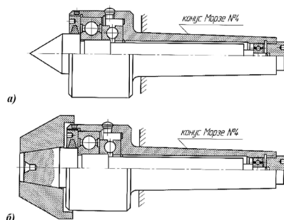
Рис. 2.14. Типы вращающихся задних центров: а) прямой; б) обратный
