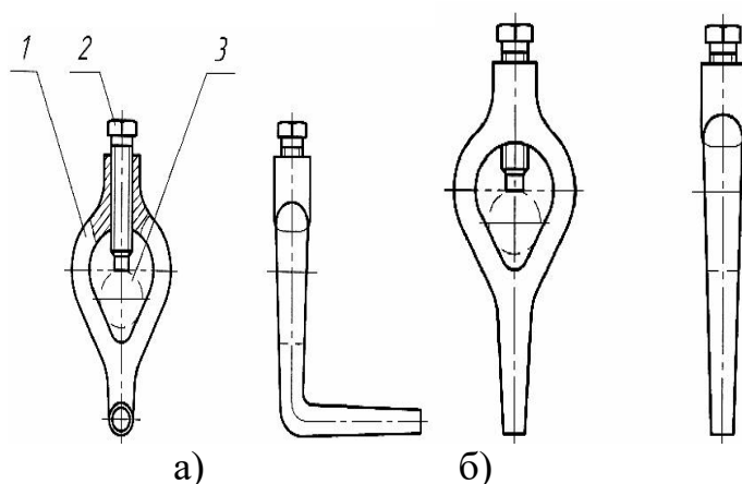
Рис. 2.6. Типы токарных хомутиков: а) с отогнутым хвостовиком; б) с прямым хвостовиком. 1– корпус хомутика; 2– винт; 3– заготовка инструмента
