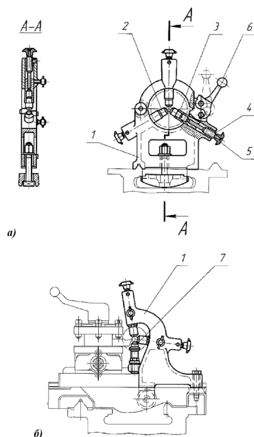
Рис. 2.15. Типы токарных люнетов: а) неподвижный; б) подвижный. 1– корпус; 2– кулачок; 3– пиноль; 4– винт; 5– рукоятка; 6– ручка зажима; 7– домкратик
