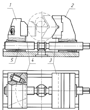
Рис. 3.1. Универсальные самоцентрирующие переналаживаемые тиски
