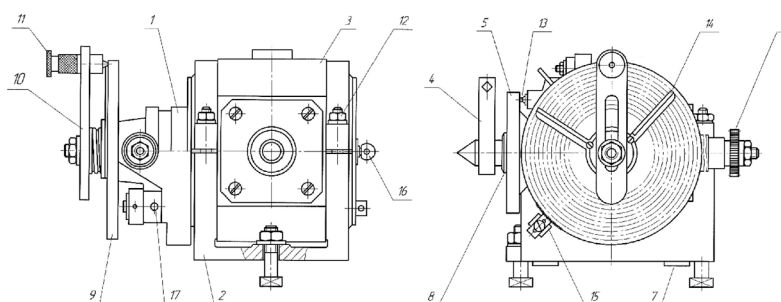
Рис. 3.2. Универсальная делительная головка
