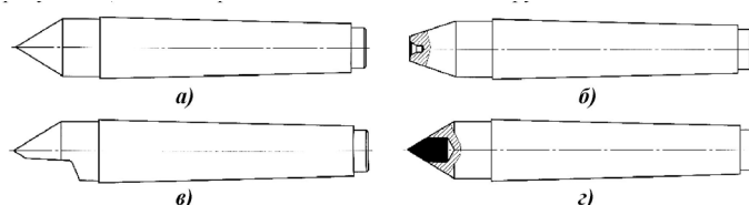
Рис. 2.13. Типы невращающихся задних центров: а) жесткий центр; б) обратный центр; в) полуцентр; г) твердосплавный центр
