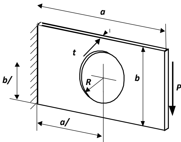
Рис. 2.1.1 Рассматриваемая конструкция
