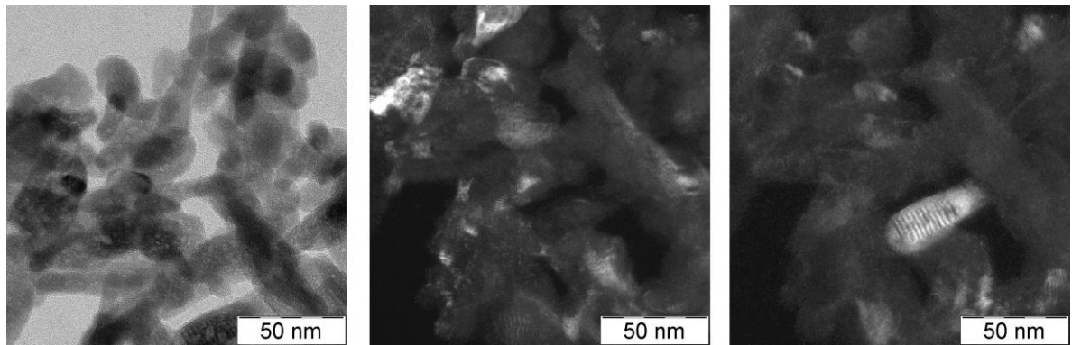
Рис. 1 Светлопольное и темнопольные изображения порошка гидроксиапатита
