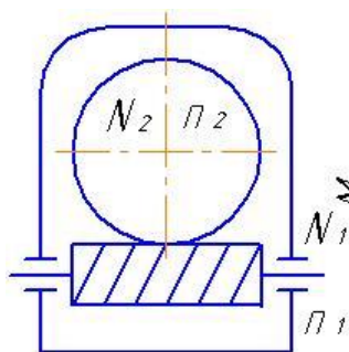
Рис. 4 Схема редуктора
