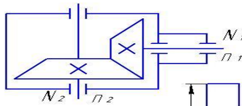
Рис. 2 Схема редуктора
