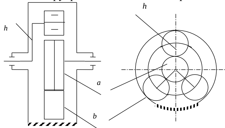
Рис. 6 Схема редуктора
