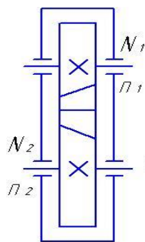
Рис. 3 Схема редуктора
