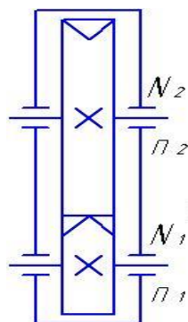
Рис. 5 Схема редуктора
