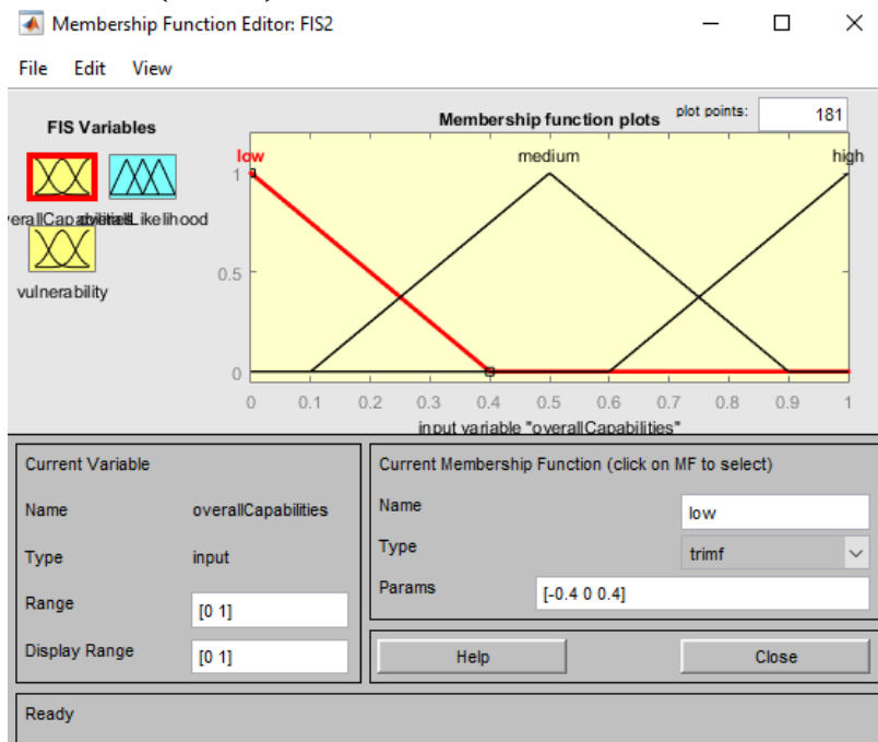
Рисунок 14 – Функции принадлежности входной переменной «средняя возможность»
