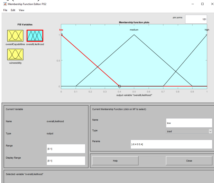
Рисунок 16 – Функции принадлежности выходной переменной «средняя вероятность»
