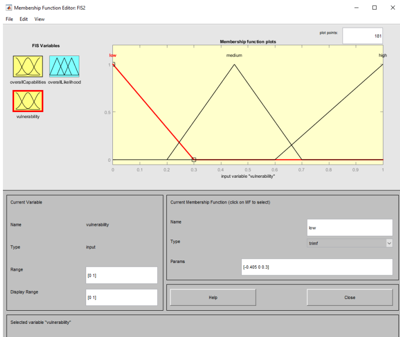
Рисунок 15 – Функции принадлежности переменной «оценка уязвимости»
