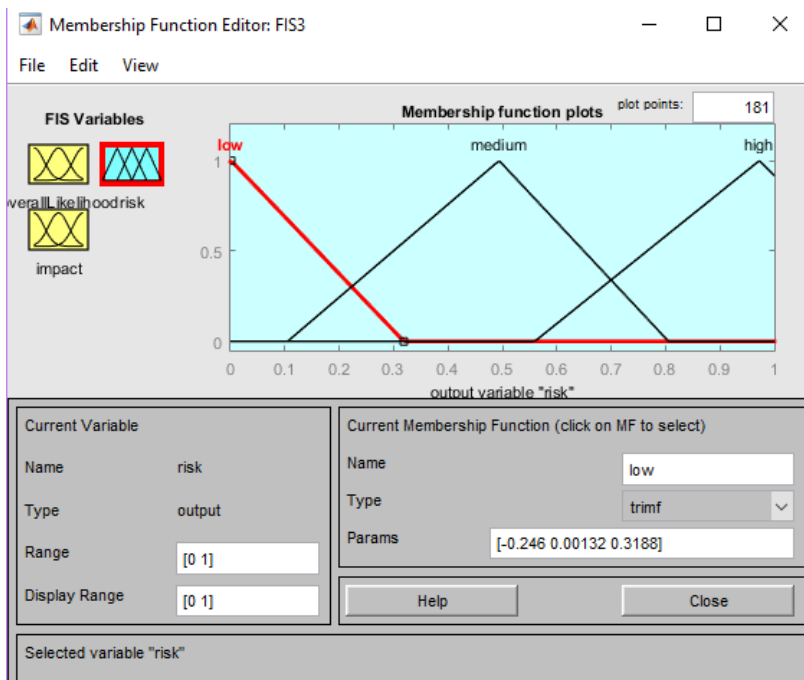
Рисунок 21 – Функции принадлежности «риск»
