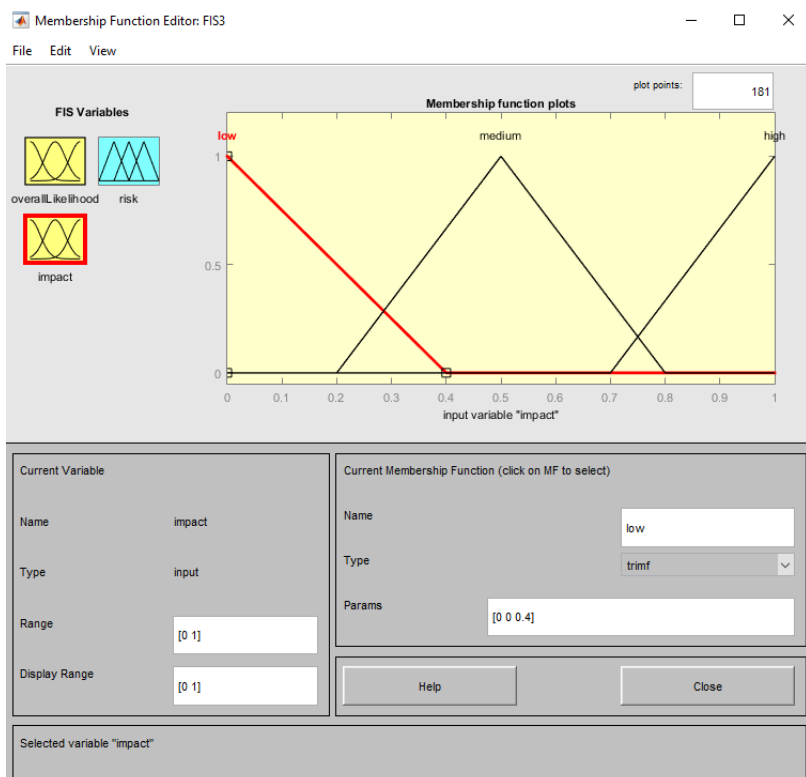
Рисунок 20 - Функции принадлежности переменной «оценка последствий»
