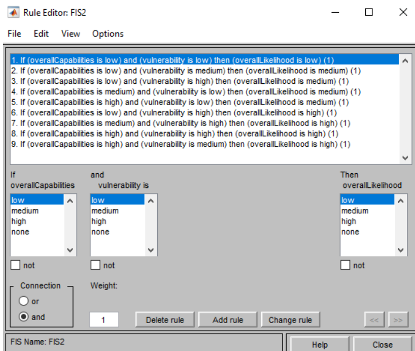
Рисунок 17 – Набор правил FIS2
