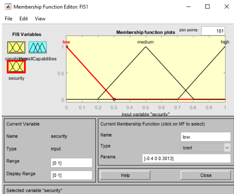
Рисунок 11 – Функции принадлежности переменной «защищенность системы»
