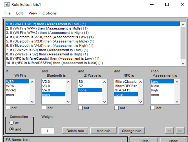
Рис.3 Настройка решающих правил Wi-Fi протокол WEP.
