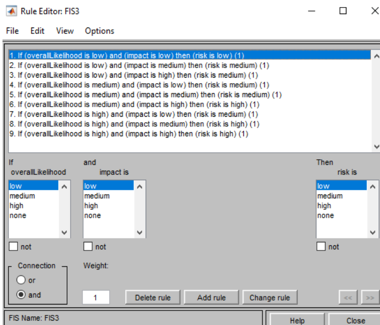
Рисунок 22 - Набор правил FIS3
