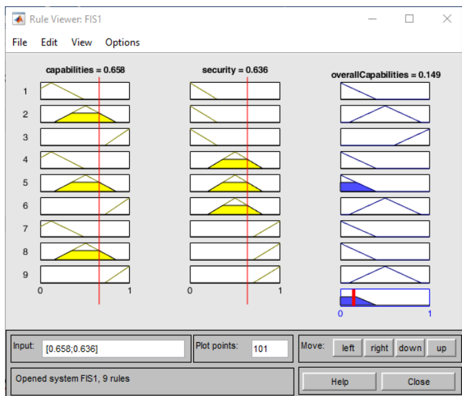
Рисунок 23 – Первый нечеткий интерфейс
