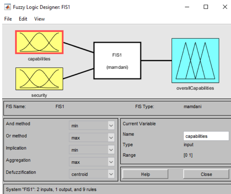
Рисунок 9 – Окно создания первого нечеткого интерфейса
