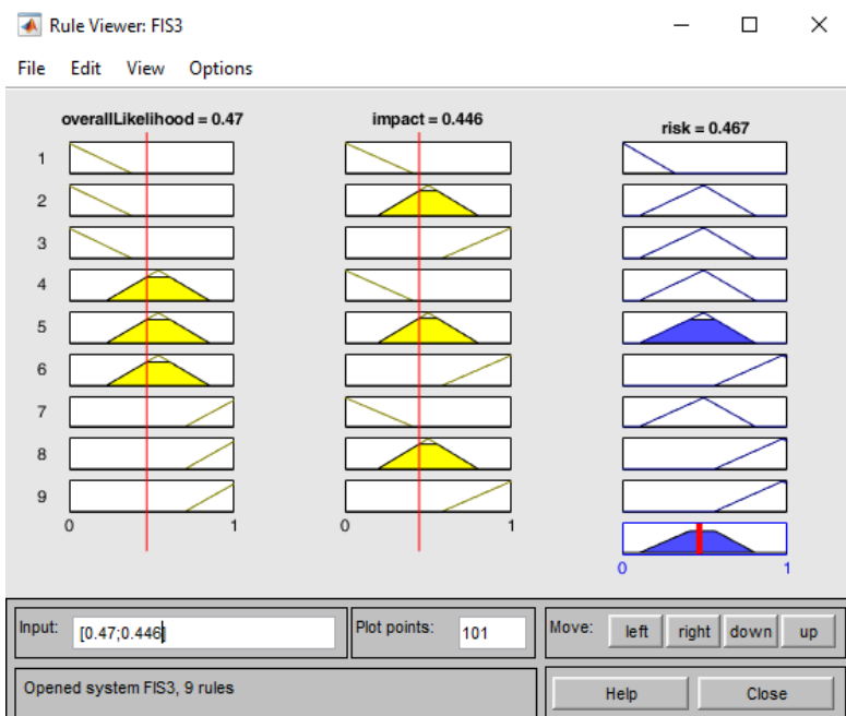
Рисунок 25 – Третий нечеткий интерфейс
