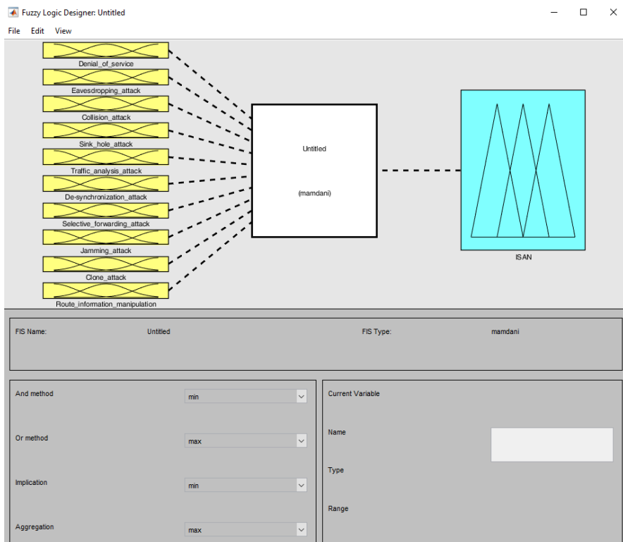
Рисунок 26 – Выходные и выходные параметры.
