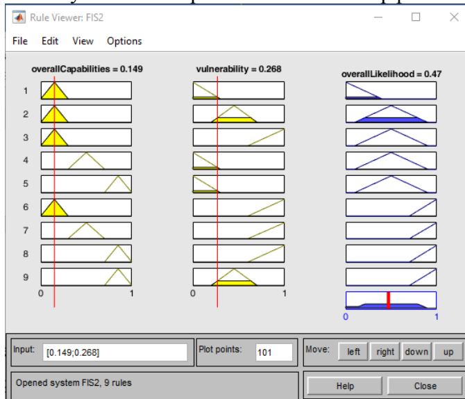
Рисунок 24 – Второй нечеткий интерфейс
