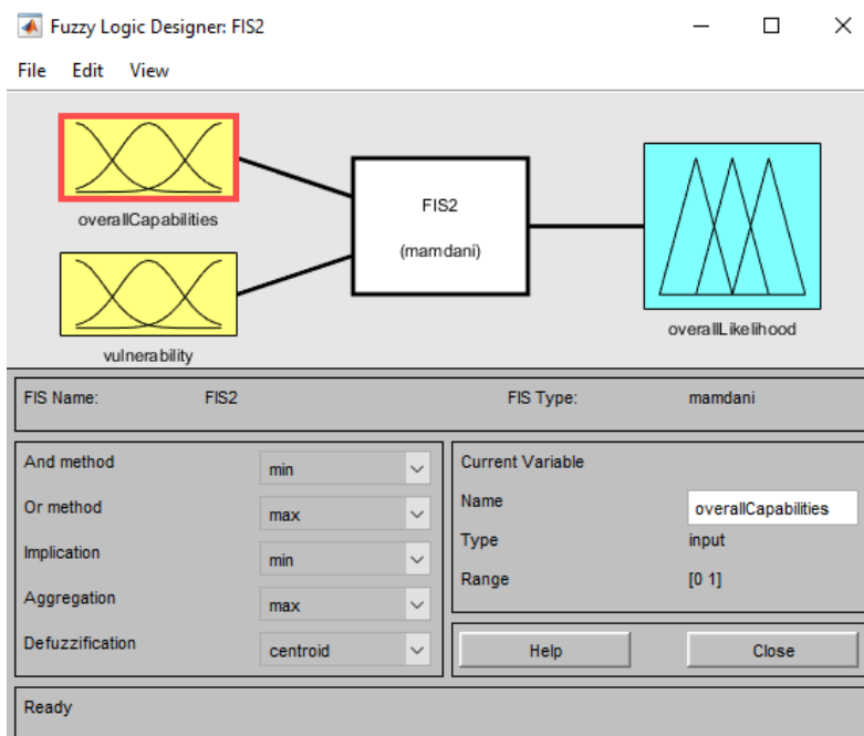
Рисунок 13 – Второй нечеткий интерфейс
