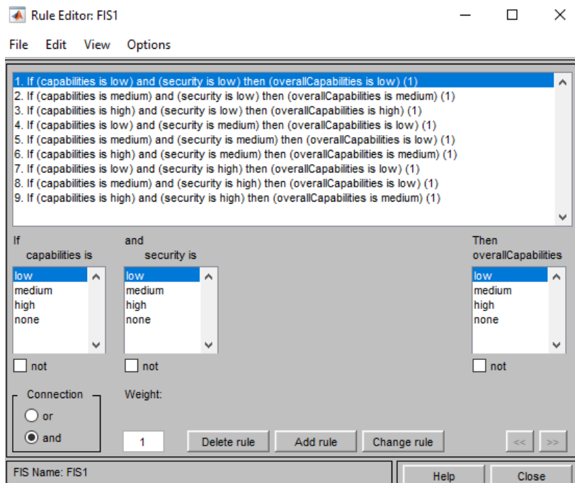
Рисунок 12 – Набор правил для FIS1
