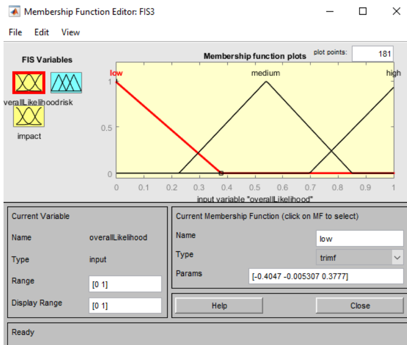
Рисунок 19 - Функции принадлежности входной переменной «средняя вероятность»
