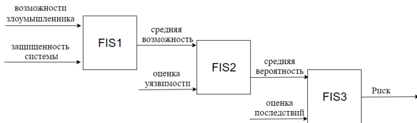
Рисунок 8 – Нечеткий алгоритм оценки риска
