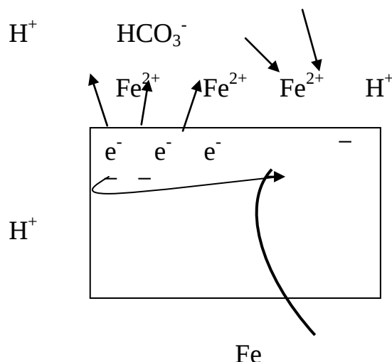
Схема электрохимической коррозии железа в кислой среде
