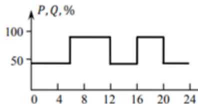
Рис. 2 График нагрузки
