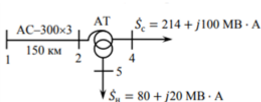
Рис.1 Схема сети
