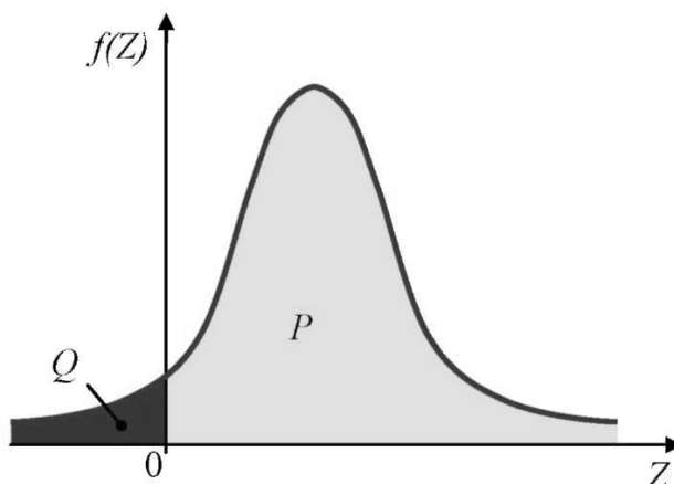
Рисунок. Распределение запаса прочности
