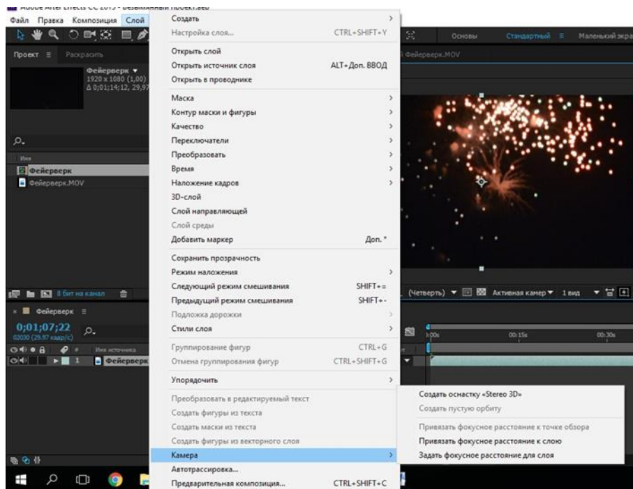
Рис. 22. Слой Камера
