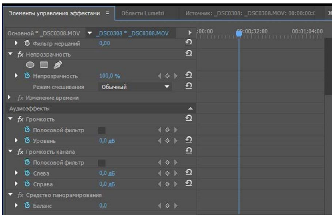
Рис. 19. Изменение громкости
