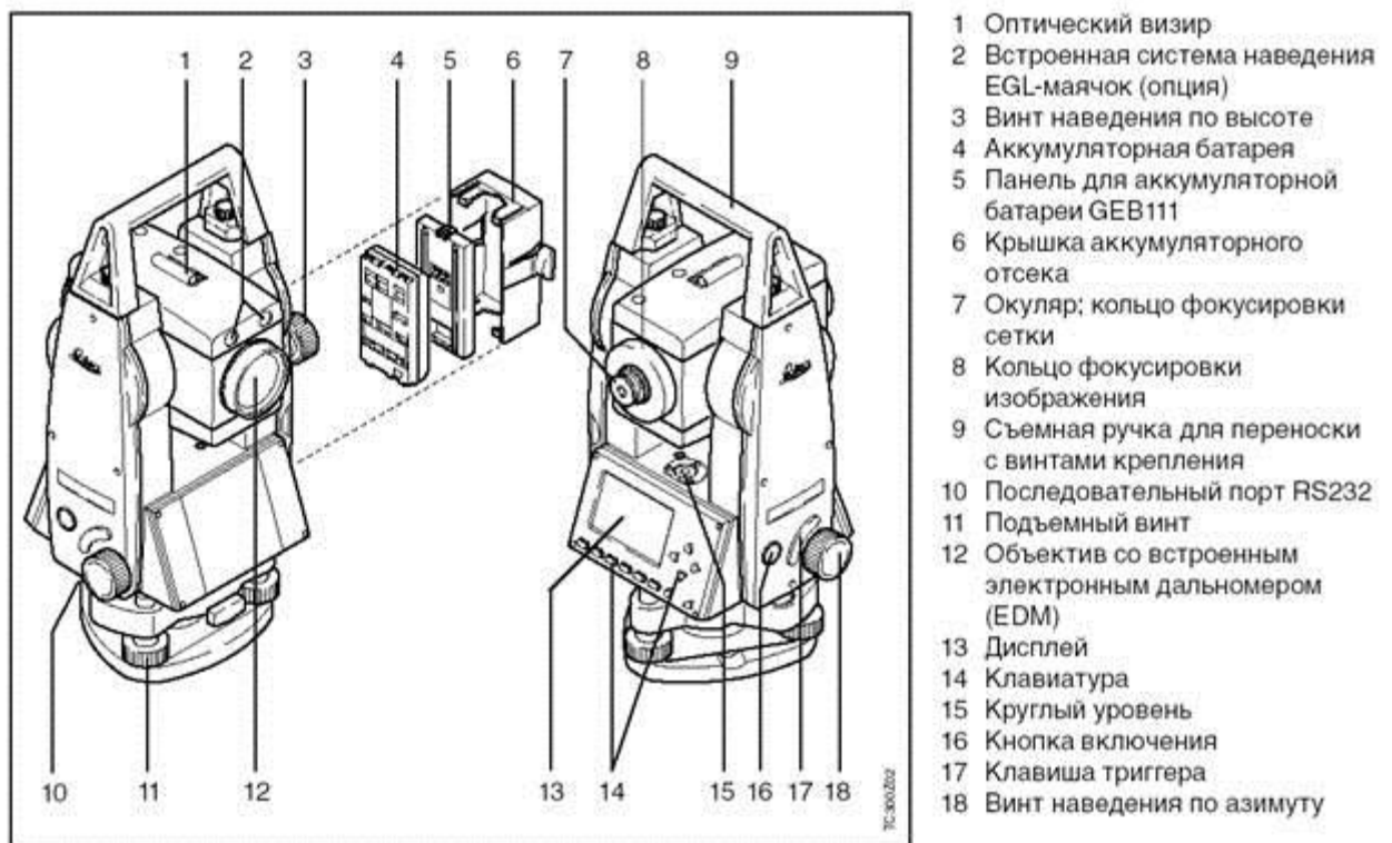
Рис. 2. Основные компоненты электронного тахеометра
