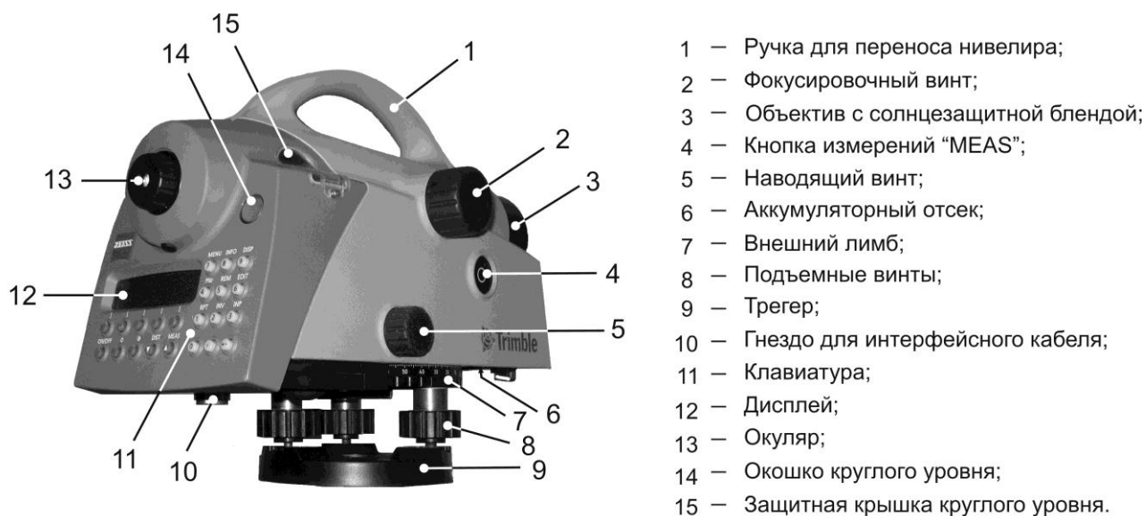
Рис. 34. Общий вид цифрового нивелира DiNi 12
