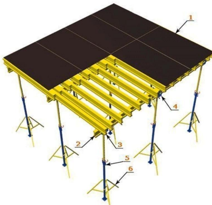
Рис. 25. Схема расстановки опалубочной системы:
