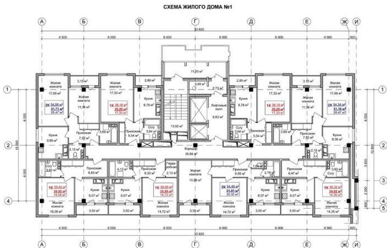
Рис. 19. План жилого дома
