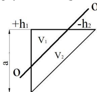
Рис. 8. Схемы определения смешанных объемов по методу трёхгранных призм.
