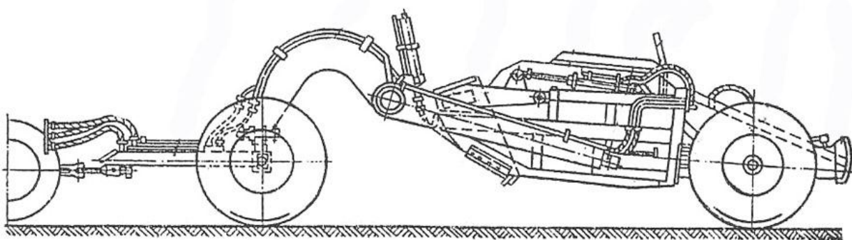
Рис. 13. Конструкция скрепера ДЗ-20
