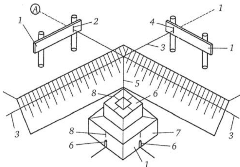
Рис. 23. Геодезическая разбивка столбчатых фундаментов: 1 — обноска; 2,8 — риски; 3 — проволока; 4 — положение разбивочных осей на обноске; 5 — отвес; 6 — колышки-фиксаторы; 7 — фундамент
