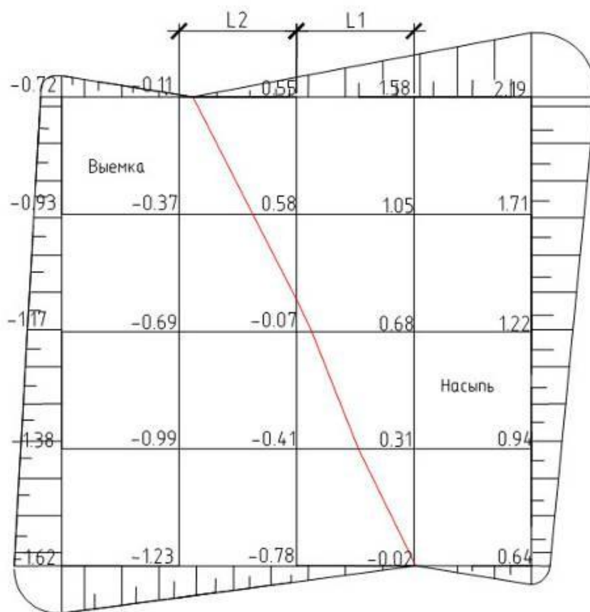
Рис. 9. Схема расчета откосов: план площадки
