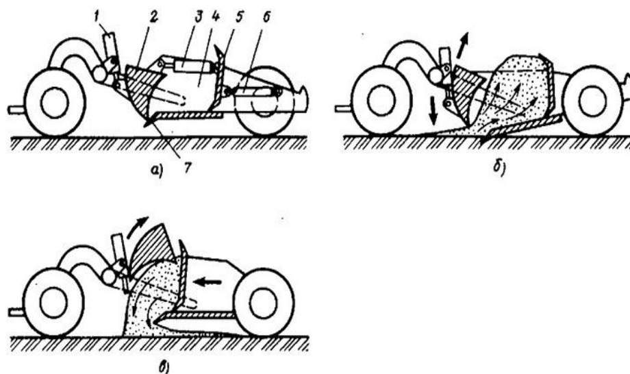
Рис. 15. Схема работы прицепного скрепера:
