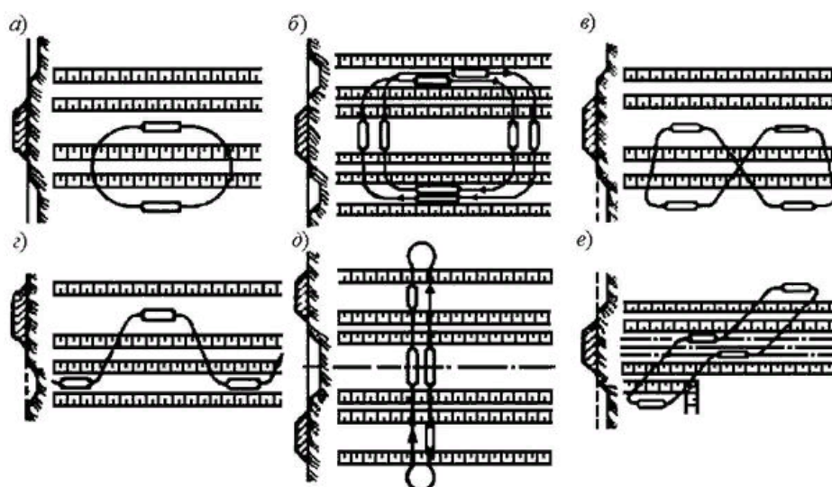
Рис. 16. Схема движения скреперов:
