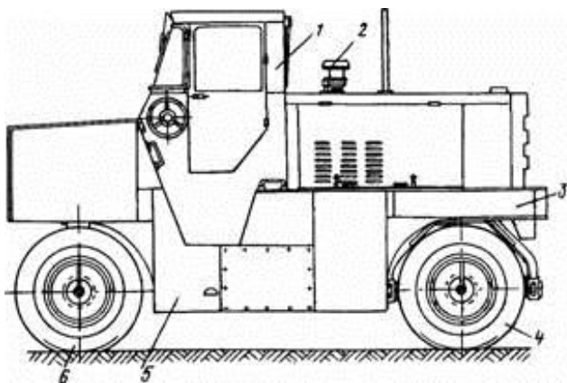
Рис. 14. Пневмоколесный каток ДУ-31А
