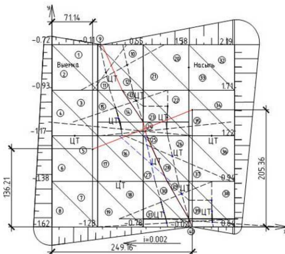
Рис. 10. Графическое определение центра тяжести элементарных фигур на планируемой площадке (ЦТ) и средней дальности перемещения грунта ( L_{ср} с координатами – ВН): нахождение центра тяжести прямоугольника (а); трапеции (б); треугольника (в)
