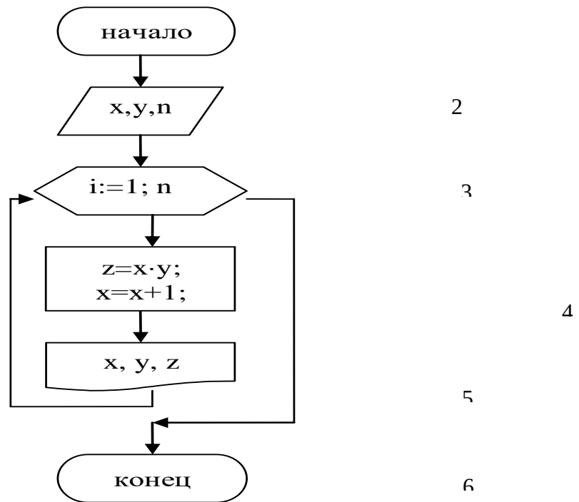
Рис.4 . Циклический алгоритм со счётчиком циклов
