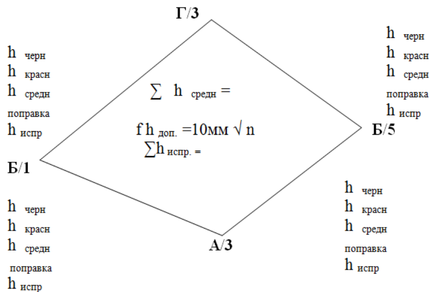
Рис. 15. Схема уязки превышений
