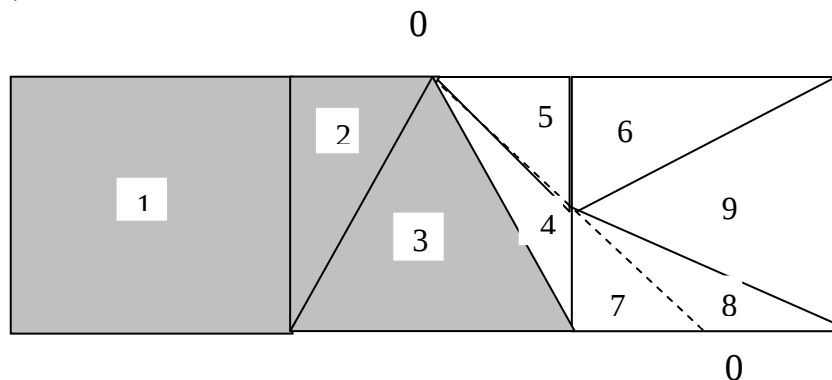
Рис. 19. Картограмма земляных работ при проектировании горизонтальной площадки (фрагмент)
