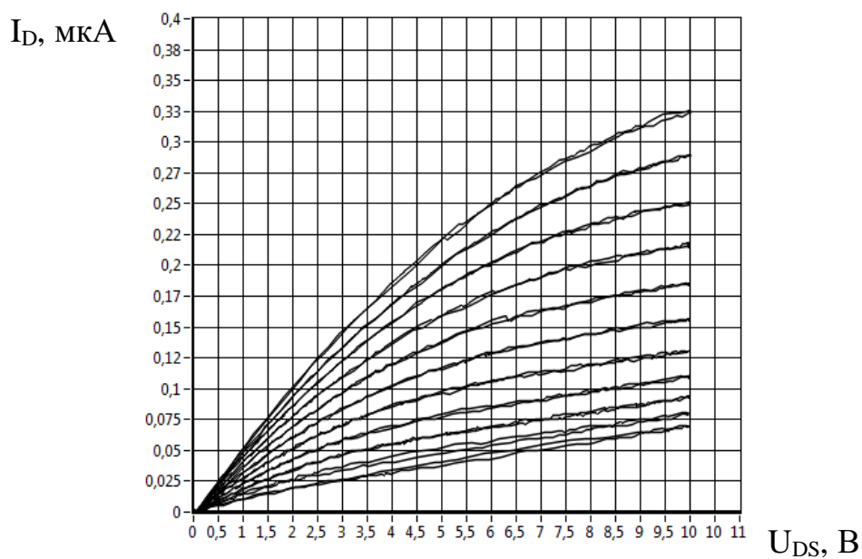
Рисунок Б.2 – ВАХ ТТФТ, измеренная на лабораторном стенде
