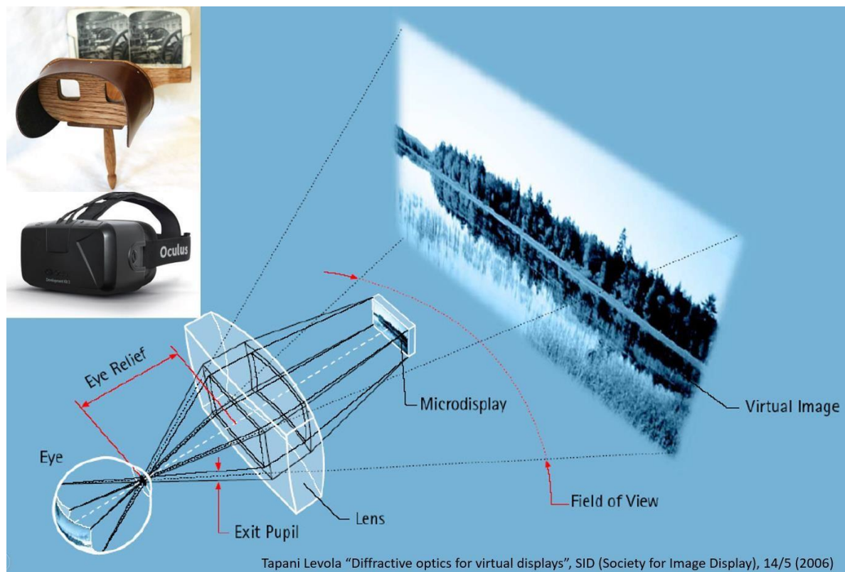
Рис. 1. Принцип работы носимых устройств виртуальной реальности
