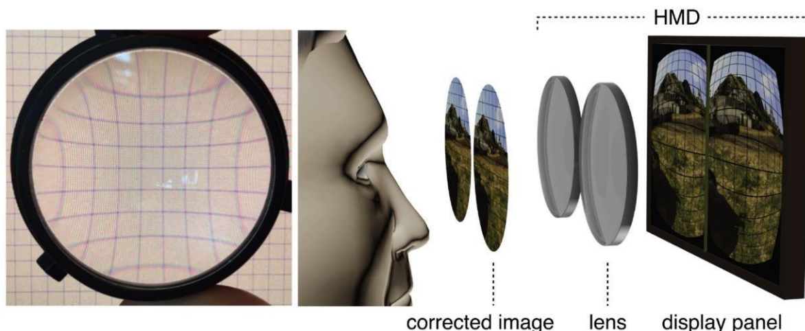
Рис. 9. Дисторсия и исправление дисторсии в очулярах систем виртуальной реальности
