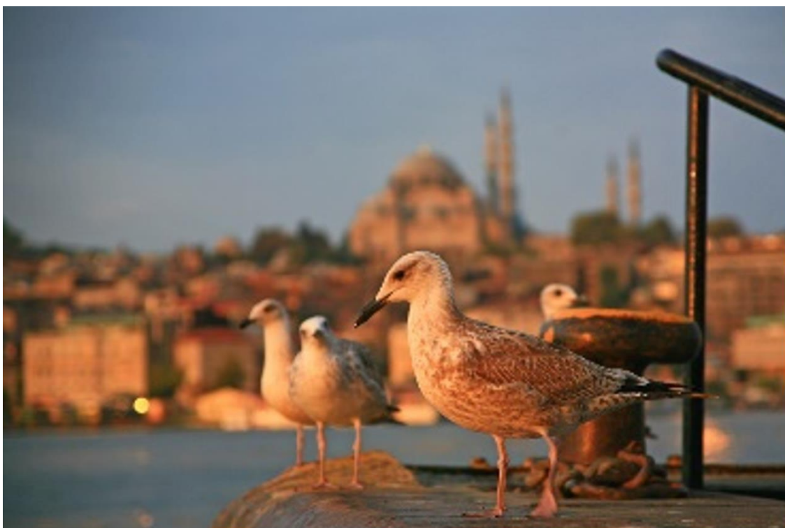
Рис. 12. Эффект аккомодации человеческого зрения
