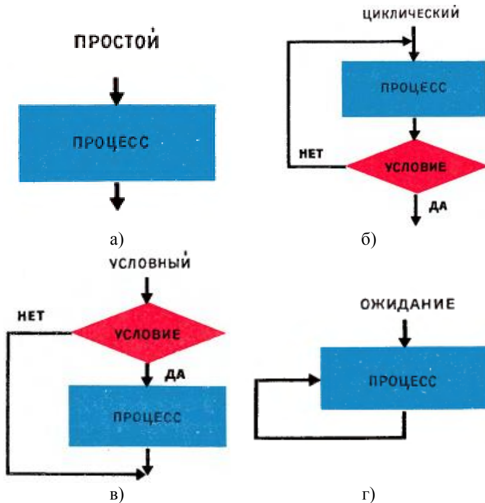
Рис. 4. Базовые процессы, происходящие в ЭВМ
