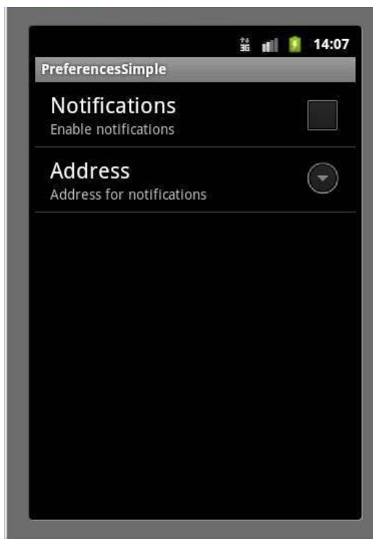
Рис.6.1. Интерфейс приложения
