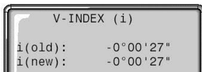
Рис. 26. Значения места зенита (предыдущее и вычисленное по новым измерениям)
