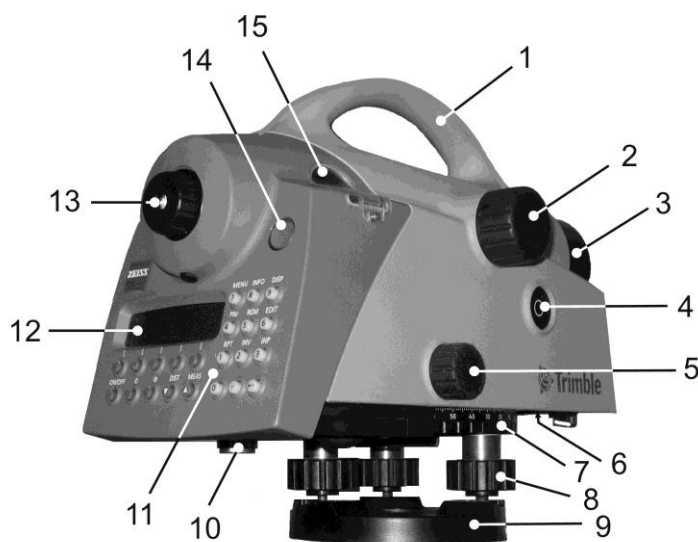
Рис. 34. Общий вид цифрового нивелира DiNi 12
