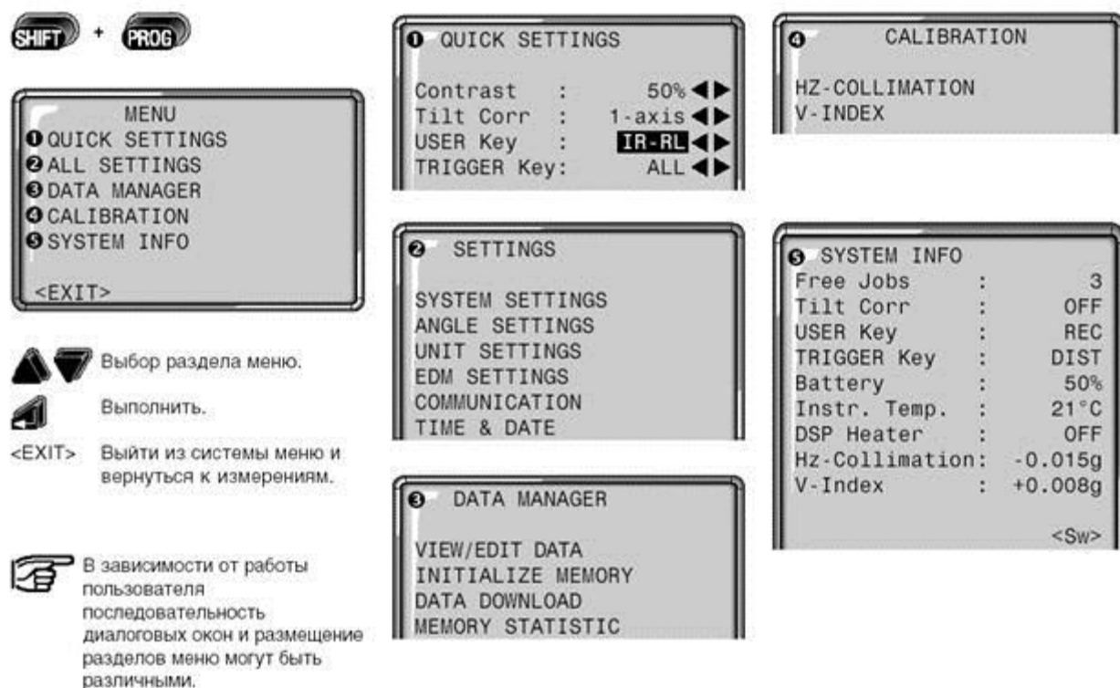
Рис. 5. Структура меню программного обеспечения TC307
