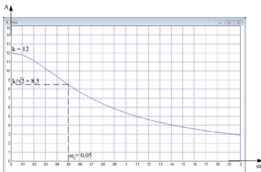
Рис. 5. АЧХ апериодического звена с параметрами k=12 и T=20 сек
