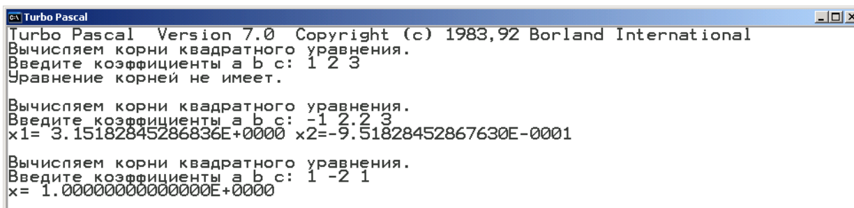
Рис.1. Программная реализация разветвляющегося алгоритма с использованием оператора if
