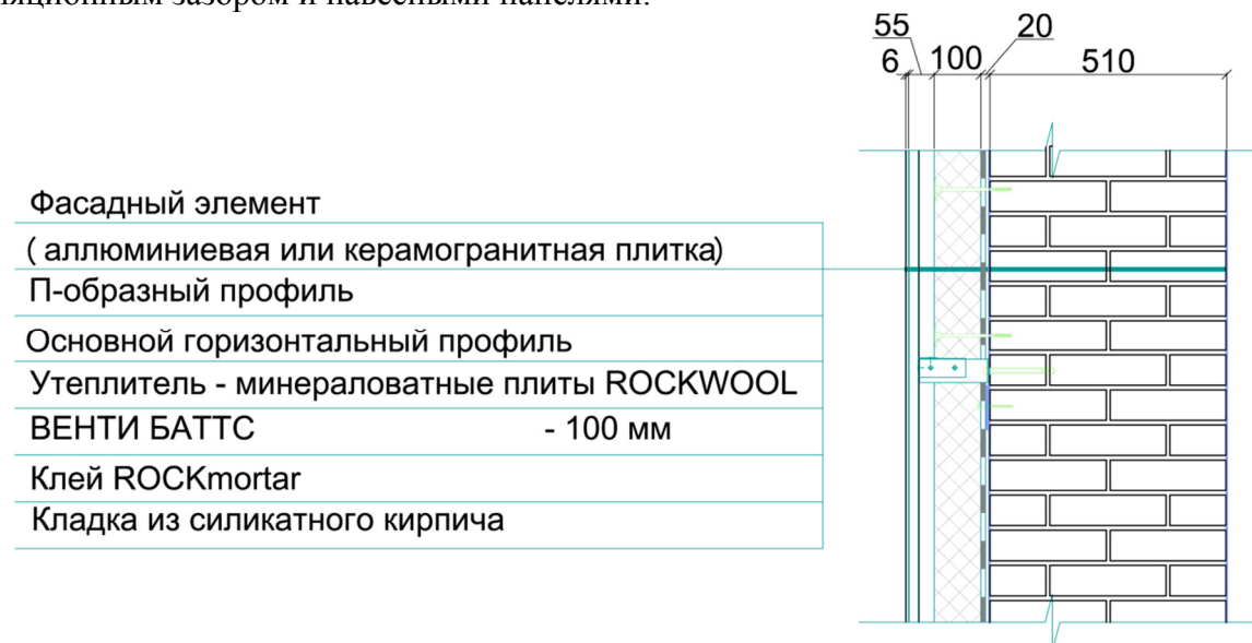
Рис. 7.1. Фрагмент навесного вентилируемого фасада дома.
