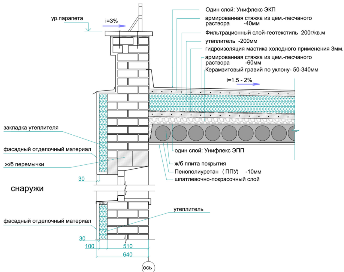
Рис. 7.3. Узел плоской кровли с парапетом.
