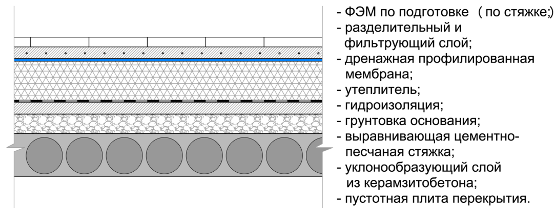
Рис. 7. 4. Инверсионная (перевернутая) эксплуатируемая кровля.
