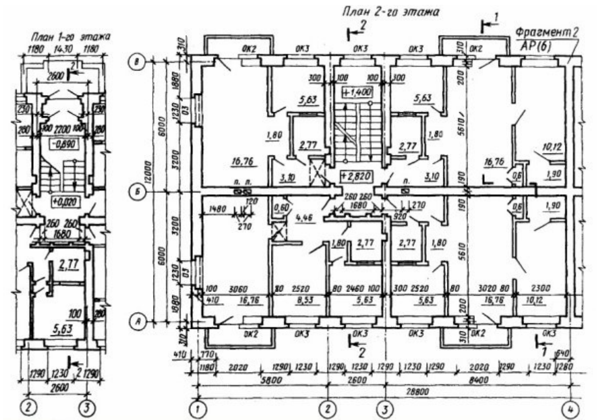
Рис. 2. Фрагмент плана типового этажа и входной группы 1-го этажа.
