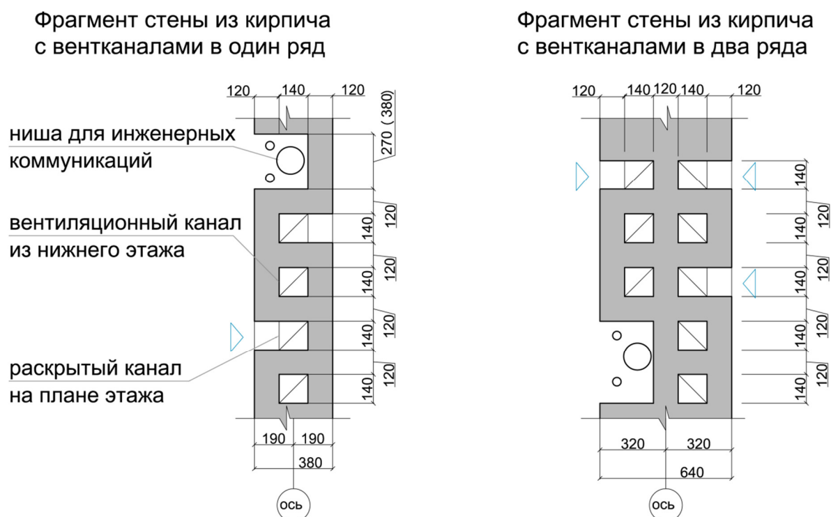
Рис. 7.2. Варианты решений вентиляционных каналов в один и два ряда.
