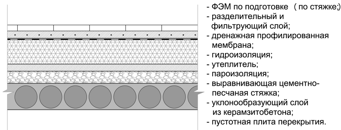
Рис. 7.3. Традиционная эксплуатируемая кровля.
