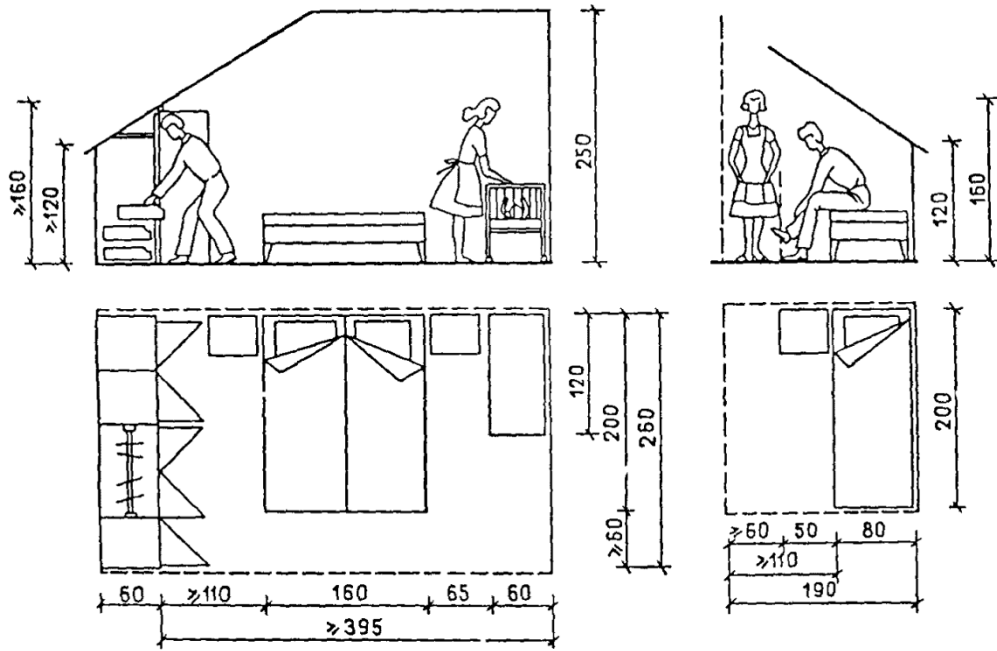
Рис. 1. Примеры использования пониженной части мансарды
