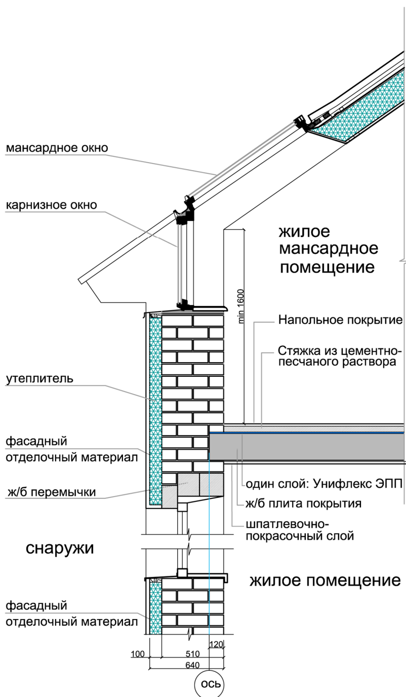
Рис. 7.6. Узел скатной кровли с окнами в мансарде.
