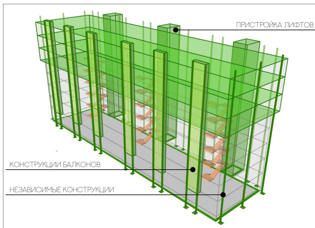
Рис.1.3. Схема реконструкции дома (способ №3)
