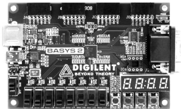
Рис. 5. Отладочная плата Digilent Basys 2
