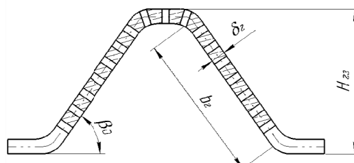
Рис. 6. Гофровый заполнитель
