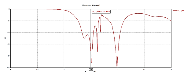
Рис. 3. S-параметры антенны
