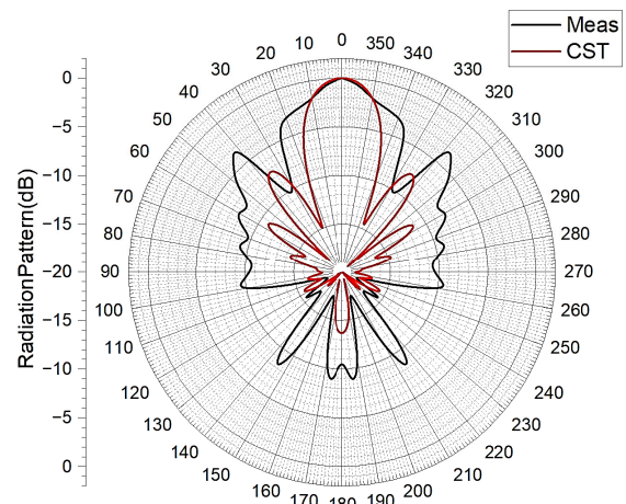
Рис. 8. Диаграммы направленности модели и макета антенной системы
