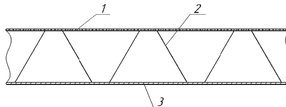
Рис. 1. Конструкция с гофровым заполнителем: 1) перфорированная обшивка; 2) гофрированный заполнитель; 3) сплошная обшивка
