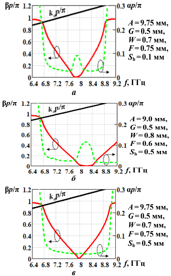
Рис. 3. Дисперсионные характеристики ЭОЛПП: а), б) при отсутствии балансировки; в) в сбалансированном состоянии
