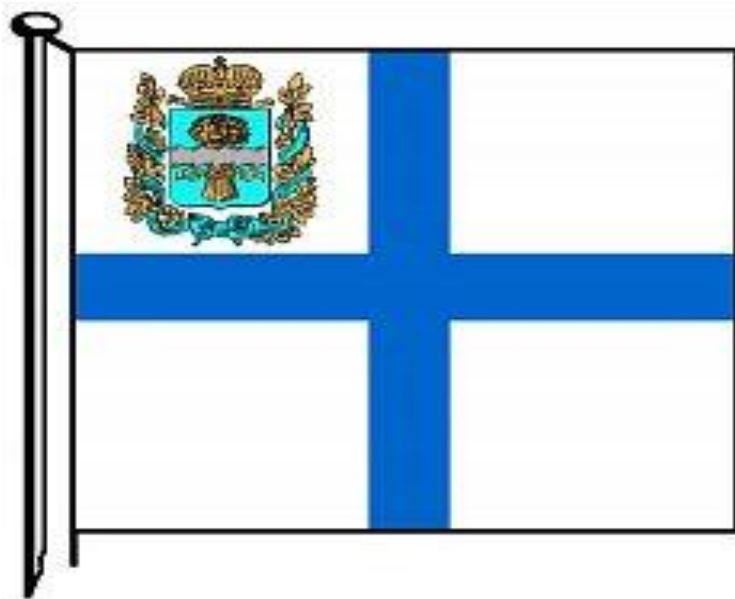
Рис. 3. Кормовой флаг
