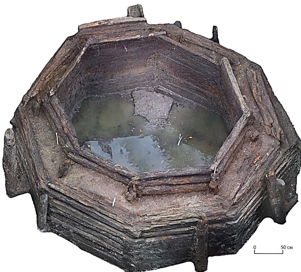
Рис. 1. Изометрическая проекция башни, обследованной в ходе раскопок в г. Усмань.
