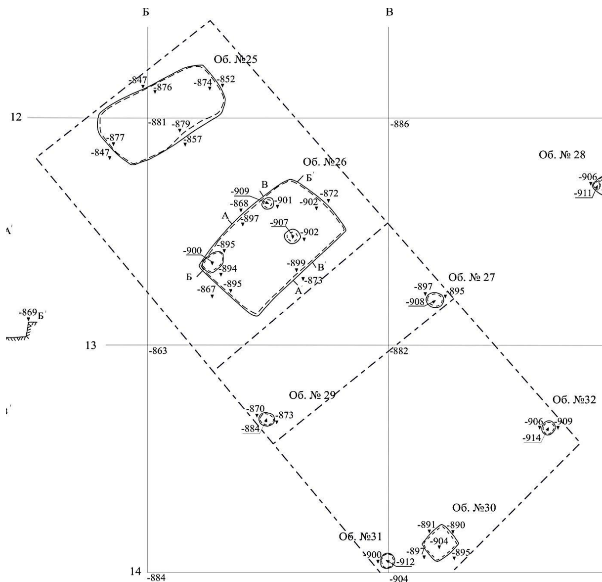
Рис. 2. План жилой постройки по матерiku.
