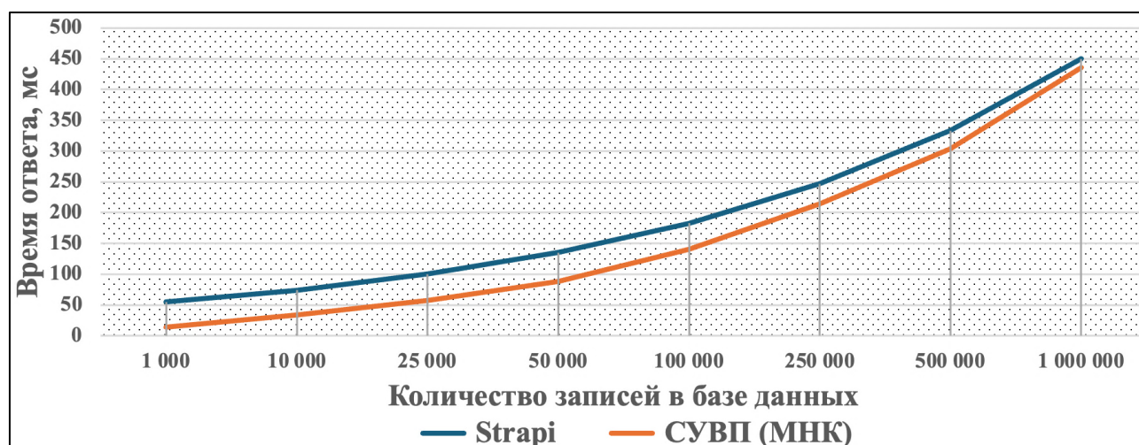
Рис. 7 – График средней скорости формирования записи в зависимости от количества строк в базе данных
