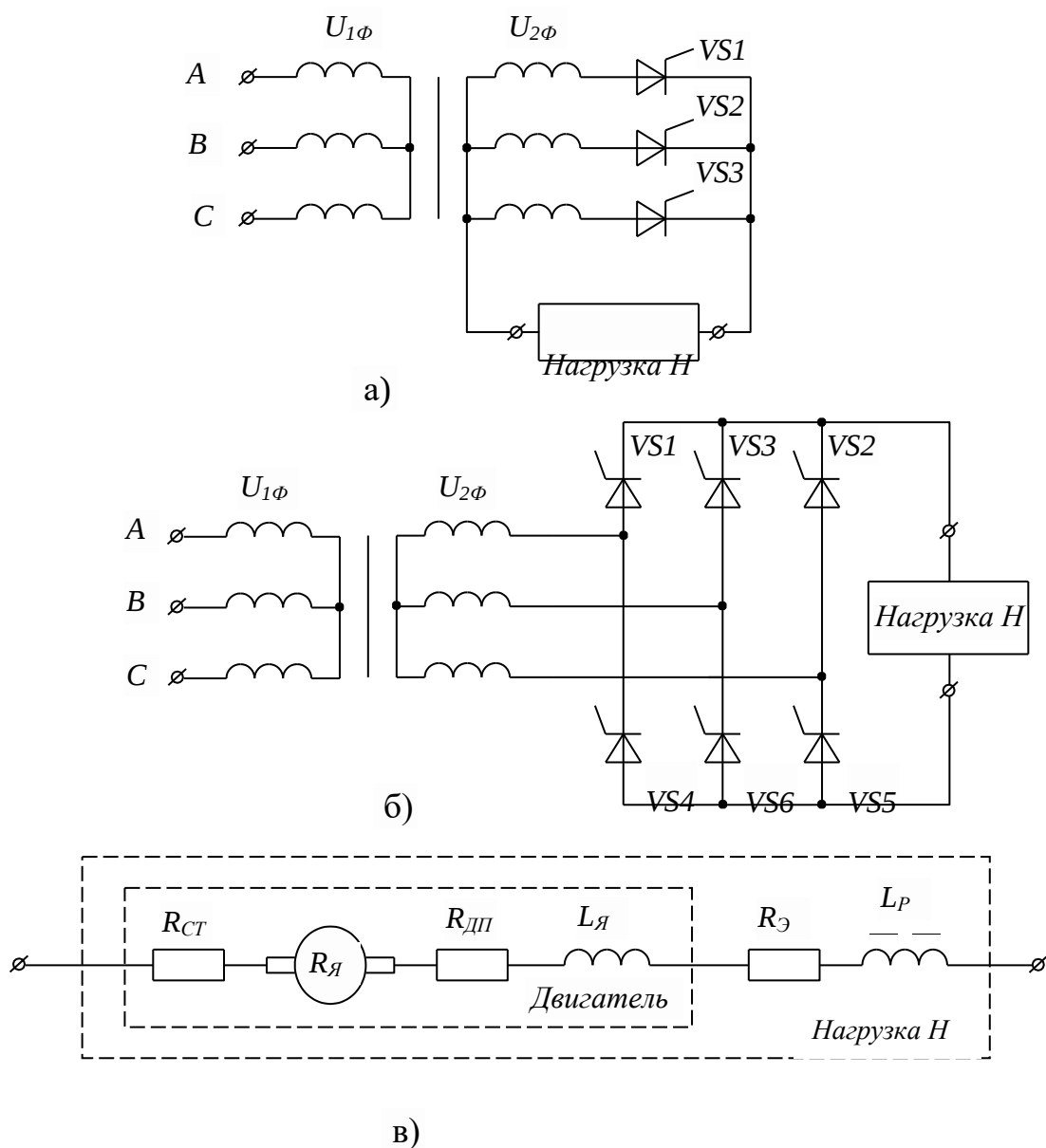
Рис. 1. Варианты схем силовых выпрямительных блоков: а – трехфазная нулевая схема; б – трехфазная мостовая схема; в – схема цепи нагрузки УВ
