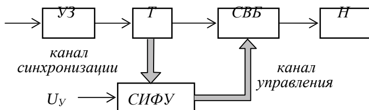
Рис. 2. Функциональная схема управляемого выпрямителя
